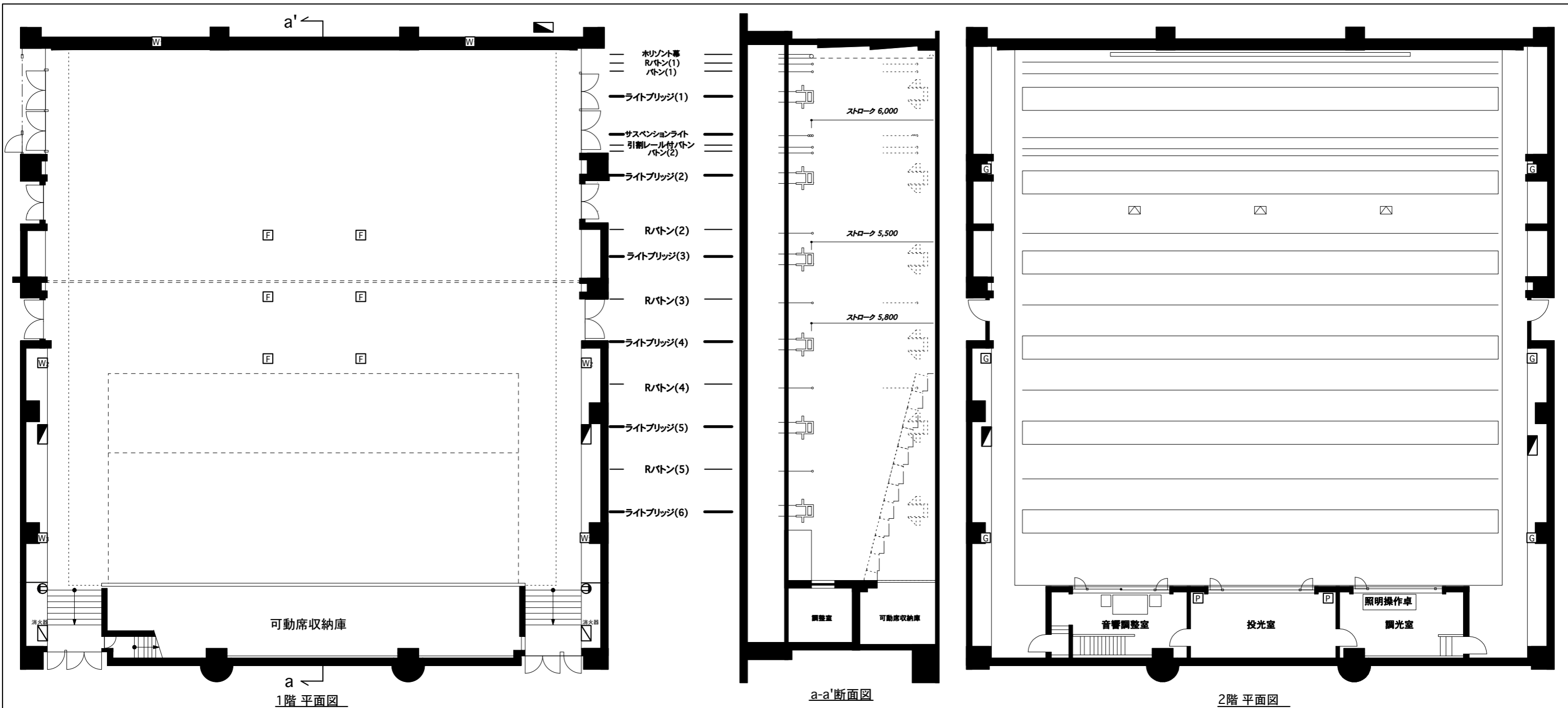
1階平面図
